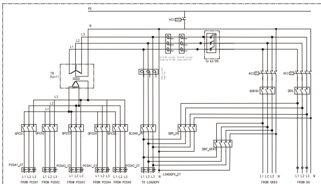
STS250D CABINET
